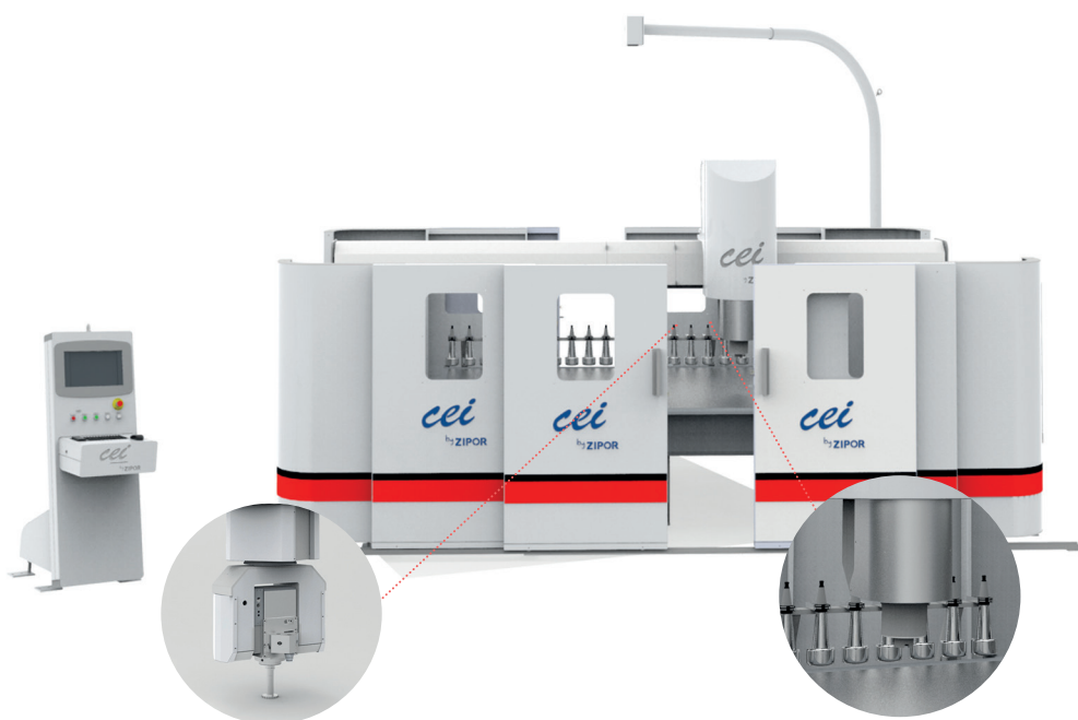
Armazém até 30 ferramentas com troca automática
